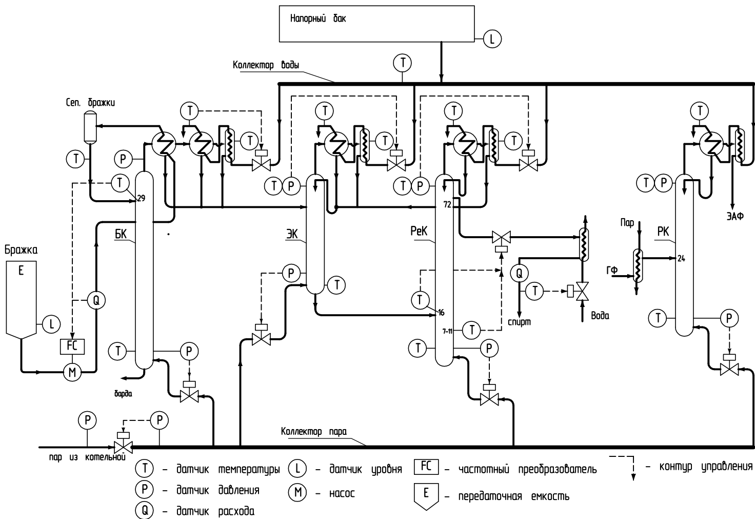
Схема автоматизации бразоректификационной установки
